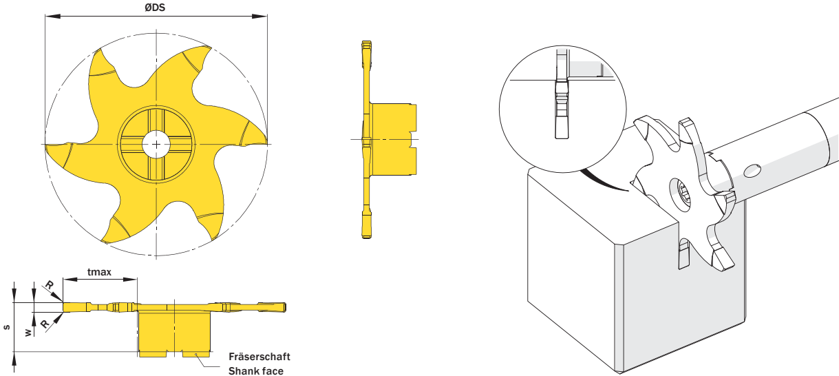
Abbildung zeigt / Drawing shows: 9W1.0120.020.28 G
